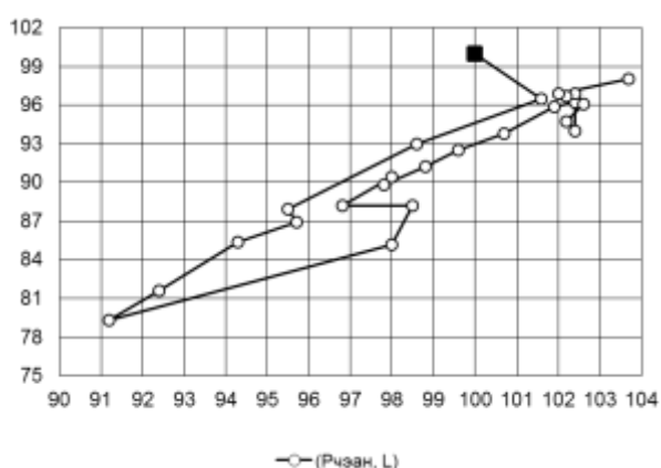
Рис. 3. График зависимости числа занятых L от численности экономически активного населения P_{чзан} ( L=F(P_{чзан}) ) в периоде с 1991 по 2015 год.
