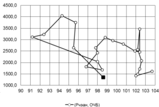
Рис. 4. График зависимости общего уровня безработицы OЧБ от численности экономически активного населения P_{чзан} ( OЧБ=F(P_{чзан}) ) в периоде с 1993 по 2015 год.
